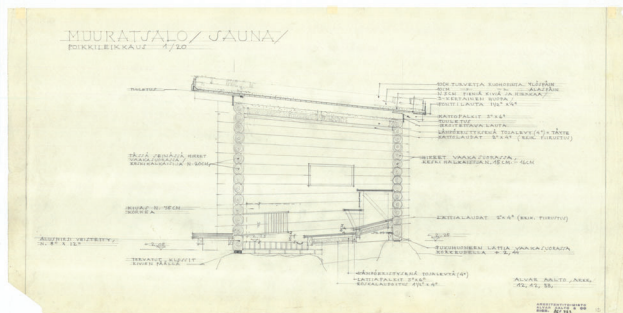
a. コエタロサウナ 断面図 アルヴァ・アアルト 所蔵: アルヴァ・アアルト財団
